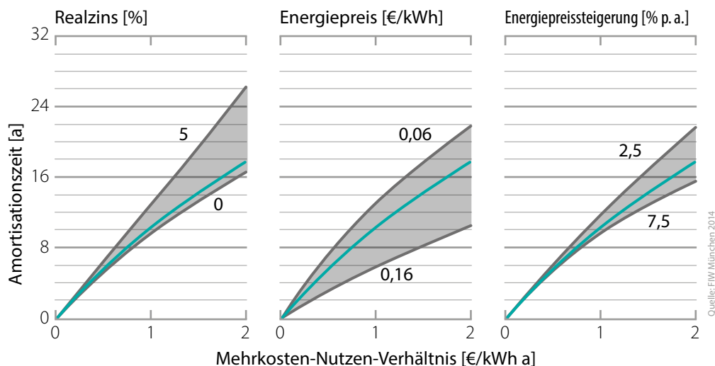
Abbildung 13: Einfluss von verschiedenen Parametern auf die Amortisationszeit unter Berücksichtigung der Schwankungsbreiten und in Abhängigkeit vom Mehrkosten-Nutzen-Verhältnis
