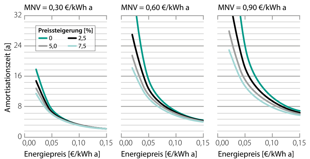
Abbildung 12: Verlauf der Amortisationszeit in Abhängigkeit vom Energiepreis in Euro pro Kilowattstunde und Jahr und von der Energiepreiserhöhung in Prozent für verschieden hohe Investitionen (Annahme: U-Wert Bestand = 1,4 W/(m 2 K); U-Wert nach Sanierung = 0,24 W/(m 2 K))
