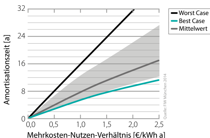
Abbildung 14: Einfluss aller Parameter nach Tabelle 5 auf die Amortisationszeit mit Angabe des Konfidenzintervalls der Monte-Carlo-Analyse und Darstellung des Worst-Case-Szenarios und des Best-Case-Szenarios in Abhängigkeit von den Investitionskosten in Euro pro Quadratmeter. Die orangefarbene Linie zeigt die mittlere Amortisationszeit.
